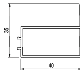
Profil pre možnosť odsadenia výrobku
