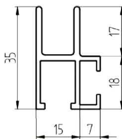
Rámový profil dvojitý
